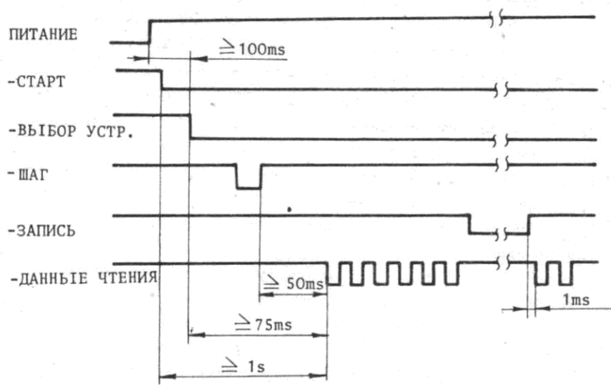
ФИГ.3 ВРЕМЯДИАГРАММА СИГНАЛОВ ПРИ ОПЕРАЦИИ "ПОИСК"
