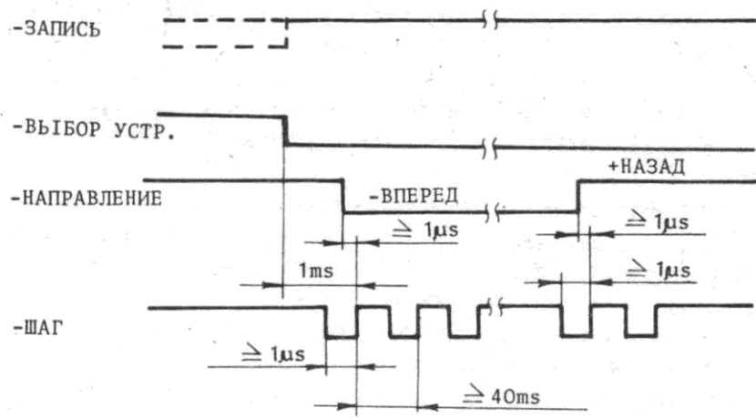
ФИГ.3 ВРЕМЯДИАГРАММА СИГНАЛОВ ПРИ ОПЕРАЦИИ "ПОИСК"
