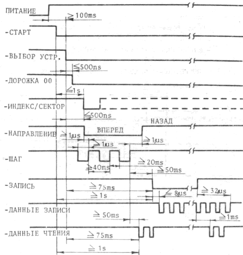
ФИГ.8 ОБОБЩЕННАЯ ВРЕМЯДИАГРАММА ИНТЕРФЕЙСНЫХ СИГНАЛОВ
