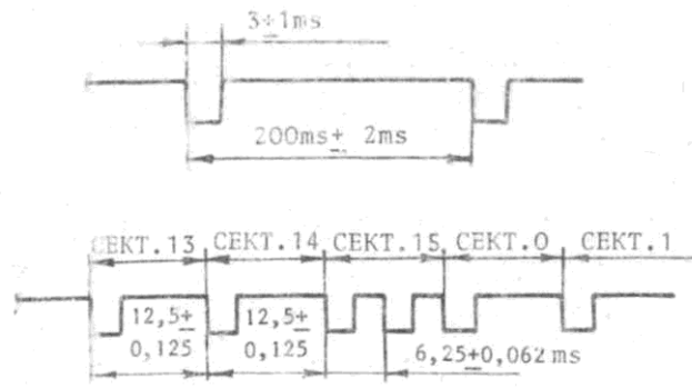
ФИГ.10 ВРЕМЯДИАГРАММА СИГНАЛА, ПЕРЕДАВАЕМОГО ПО ЛИНИИ ИНДЕКС/СЕКТОР.
